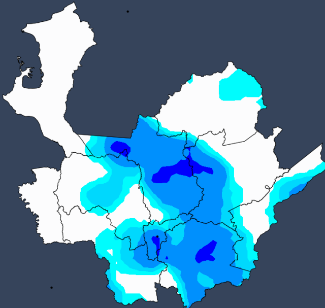
Pronóstico precipitación acumulada 24 horas, a partir de: 2020-03-23 06:00 HLC.
