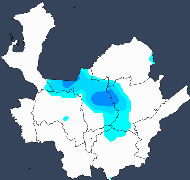
Pronóstico precipitación acumulada 06 horas, a partir de: 2020-03-22 12:00 HLC.
