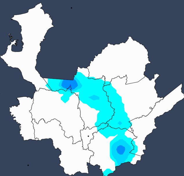
Pronóstico precipitación acumulada 06 horas, a partir de: 2020-03-22 18:00 HLC.
