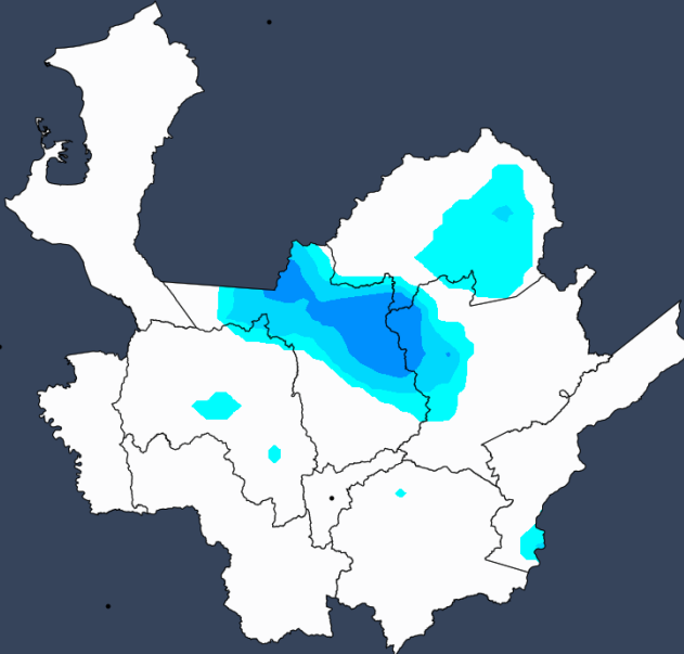
Pronóstico precipitación acumulada 24 horas, a partir de: 2020-03-22 06:00 HLC.
