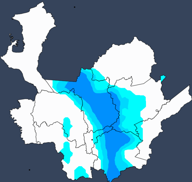
Pronóstico precipitación acumulada 06 horas, a partir de: 2020-03-21 12:00 HLC.
