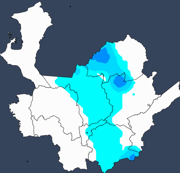
Pronóstico precipitación acumulada 06 horas, a partir de: 2020-03-21 18:00 HLC.
