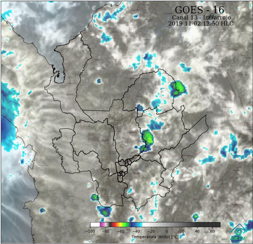
Precipitación representada en la imagen satelital IR-GOES 16 noviembre 02 de 2019 – Hora 12:50 pm.
