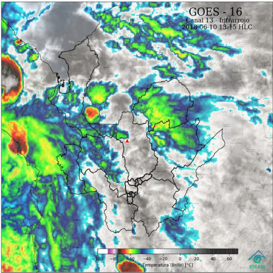
Nubosidad representada en la imagen satelital. Canal Infrarrojo - GOES 16 - IDEAM Junio 10 de 2018 - Hora 13:15 p.m.
