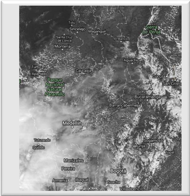
Nubosidad representada en la imagen satelital. Canal Visible – GOES - IDEAM – Diciembre 24 de 2017 – Hora 12:15 p.m. HLC.
