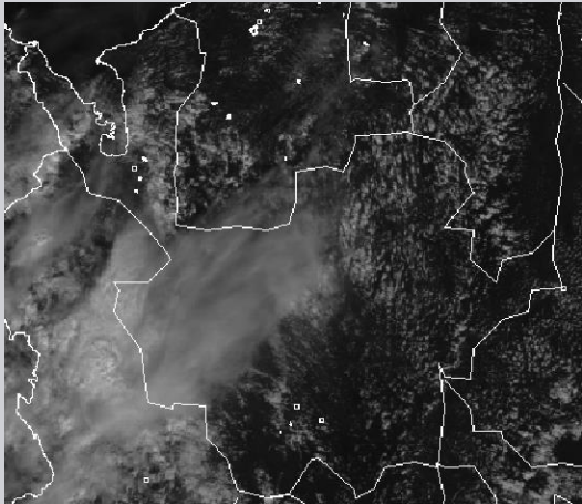
Nubosidad representada en la imagen satelital. Canal Visible – GOES- IDEAM – Diciembre 7 de 2017 Hora 11:45 a.m. HLC.
