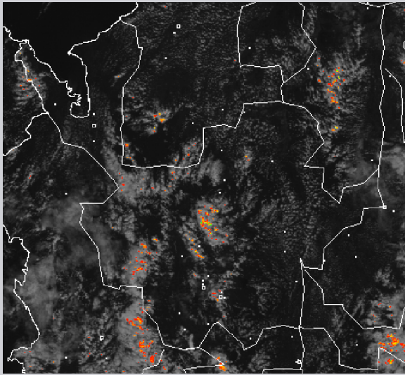
Nubosidad representada en la imagen satelital. Canal Visible GOES - IDEAM – Diciembre 10 de 2016 – Hora 12:45 p.m. HLC.
