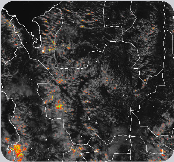
Nubosidad representada en la imagen satelital GOES. Canal Visible - IDEAM – diciembre 4 de 2016 – Hora 12:45 p.m. HLC.
