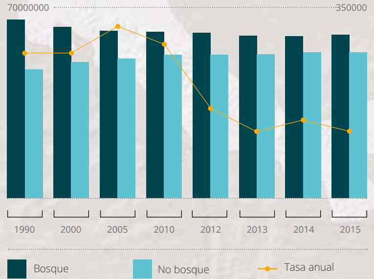
Figura 4. Dinámica de la deforestación en Colombia (1990-2015). Eje izquierdo: áreas de bosque y no bosque de 1990 a 2015. Eje derecho: tasa anual de reforestación. Fuente datos: SMBByC-IDEAM.
