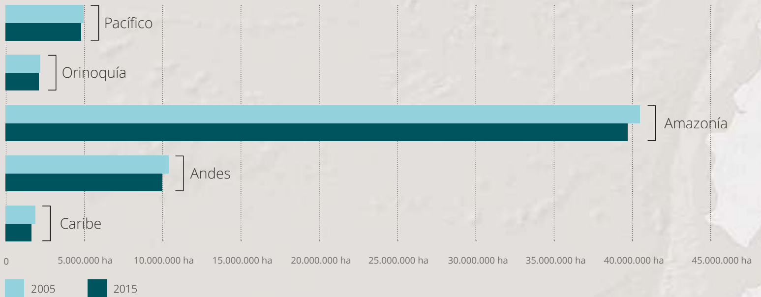
Figura 5. Cobertura de bosque natural por regiones naturales (ha). Comparación años 2005 y 2015. Fuente datos: SMBByC-IDEAM
